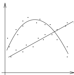
Abb. 1: Ausgleichende Gerade und ausgleichende Parabel
